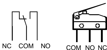
Mikrowyłączniki S1, S2, S3, S4, S5 i S6
