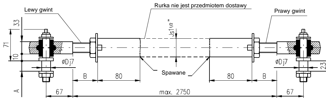
Wymiary cięgła TV 40-1/20 i TV 50-1/25
